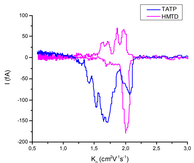
Fig. 3. Espectros en polaridad positiva y negativa de explosivos de fabricación casera analizados mediante fotoionización y DMA.
