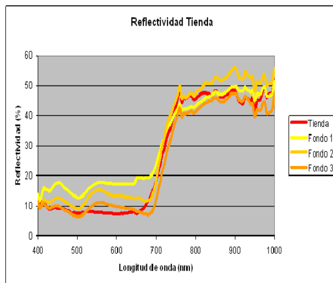
Fig. 3. a) Imagen donde se han seleccionado los diferentes fondos de la escena, junto a la muestra a caracterizar. b) Curvas de reflectancia espectral de los materiales seleccionados en la imagen.
