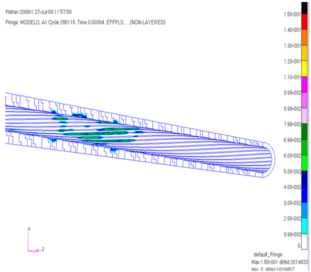
Fig. 2. Daños tras un impacto dentro del tubo.
