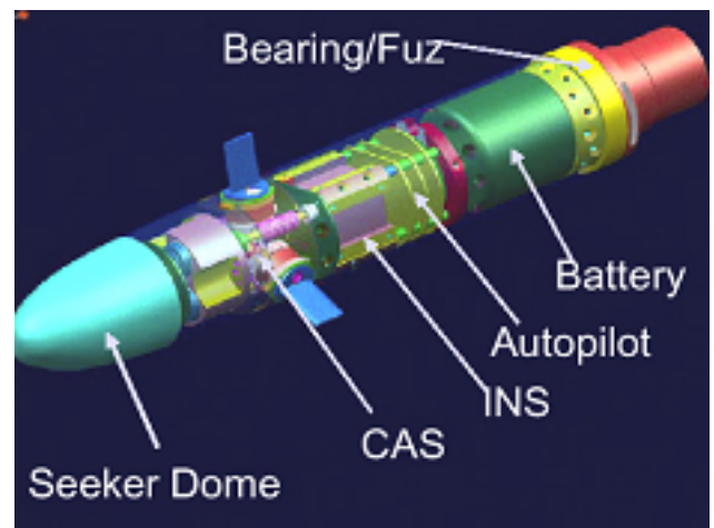
Fig. Noble LCPK. Sección de guiado
